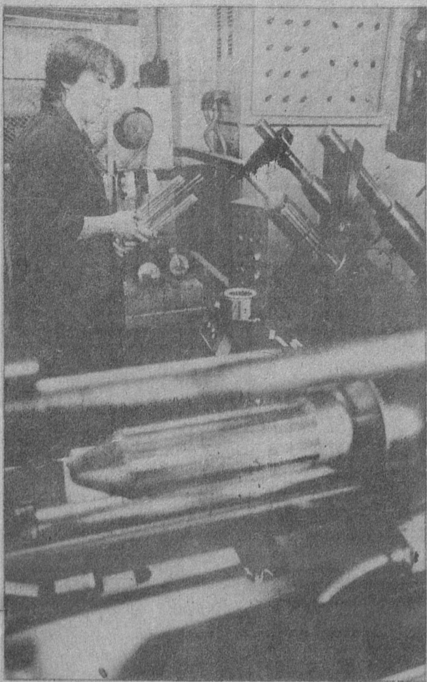
Ярославский завод «Красный маяк» приступил к промышленному производству вибратора ИВ-114, который может уплотнять бетон на глубине до 10 метров. Его предшественник делал это на глубине до 1,25 метра. Применение нового агрегата позволит намного увеличить производительность труда, улучшить качество работ.
