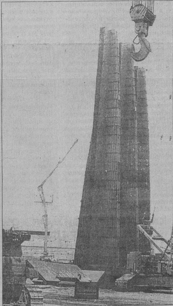
Осень, 1986. Монтаж саркофага IV блока ЧАЭС
