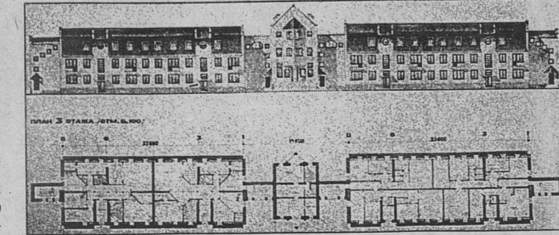
Так выглядит проект реконструкции улицы Ленинской на планшетах проектировщиков
