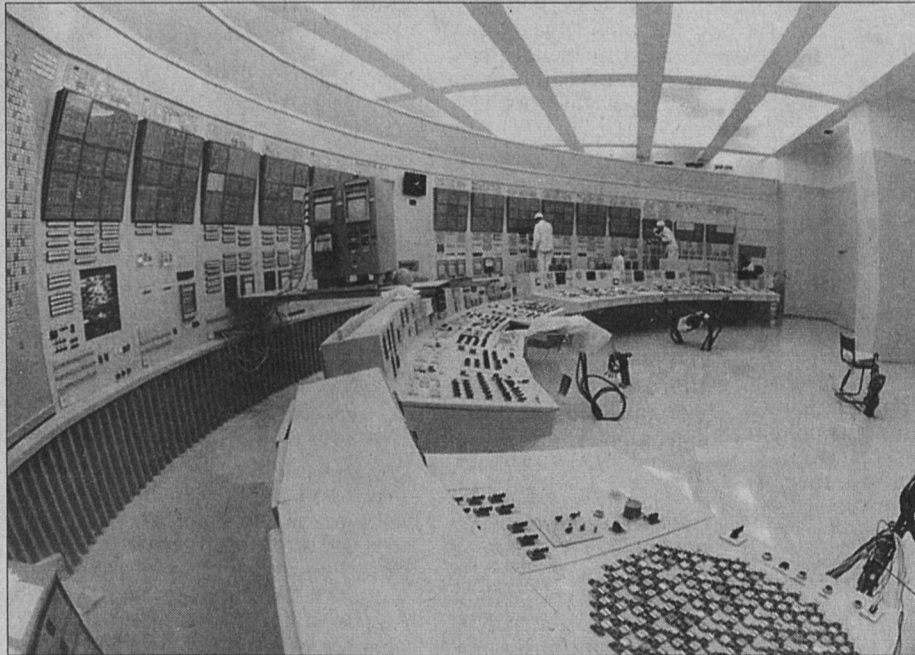
Монтаж новых приборов на блочном щите управления.
